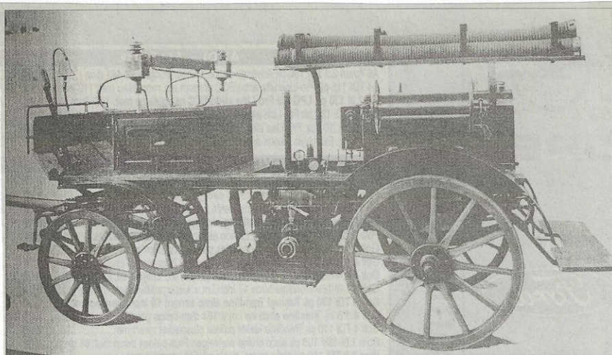
Deze vierwielige motorbrandspuit werd in 1932 door de gemeente Achtkarspelen aangekocht bij de Firma Van Bergen uit Heiligerlee. Deze firma, opgericht in 1795, was tot het eind van de 20e eeuw een gerenommeerd leverancier en fabrikant van (bronzen) brandweerpompen. Waarschijnlijk heeft een en ander te maken met het feit dat genoemd bedrijf tevens vermaard was om de fabricage van bronzen kerk- en carillonklokken. Na inruil van de oude tweewielige motorspuit was de prijs f 1150,-. Bijzonderheden van de nieuwe motorbrandspuit op vier wielen: Een 4 cilinder benzinemotor ter sterkte van 25 P.K. De pomp is een centrifugaalpomp met een capaciteit van ca. 1000 liter per minuut; spuitafstand ca. 40 meter.
